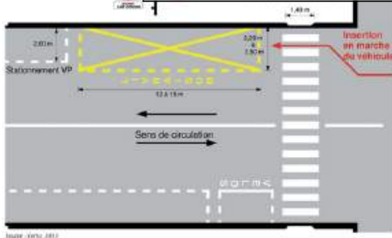
Schéma de principe d'une aire de livraison - Source : CERTU 2013 "Aires de livraison : planifier, aménager et gérer l'accueil des véhicules" - Thomas Plantier
